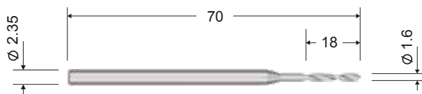
Сверло \varnothing 1.6 мм, 70 / 18 мм (Нержавеющая сталь)
