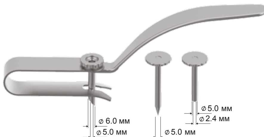
Направитель (Титановый сплав)
