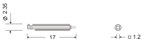
Отвертка для углового наконечника (Нержавеющая сталь)
