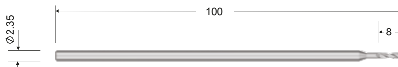
Сверло \varnothing 1.2 мм, 100 / 8 мм (Нержавеющая сталь)
