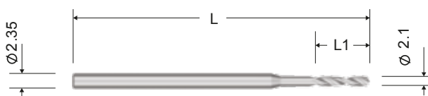
Сверло \varnothing 2.1 мм, L / L1 (Нержавеющая сталь)
