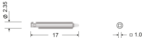
Отвертка (Нержавеющая сталь)
