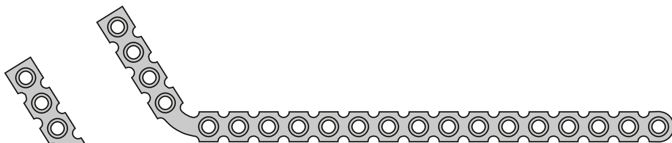
101.14 Угловая правая, 4x16 отв., правая (131 x 35 мм)
