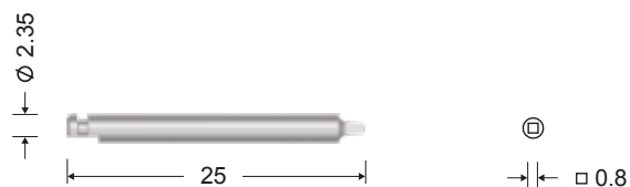
Отвертка для углового наконечника (Нержавеющая сталь)
