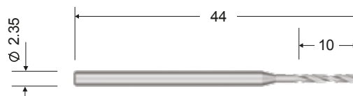
Сверло \varnothing 1.2 мм, 44 / 10 мм (Нержавеющая сталь)
