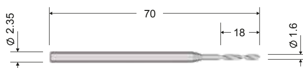
Сверло \varnothing 1.6 мм, 70 / 18 мм (Нержавеющая сталь)
